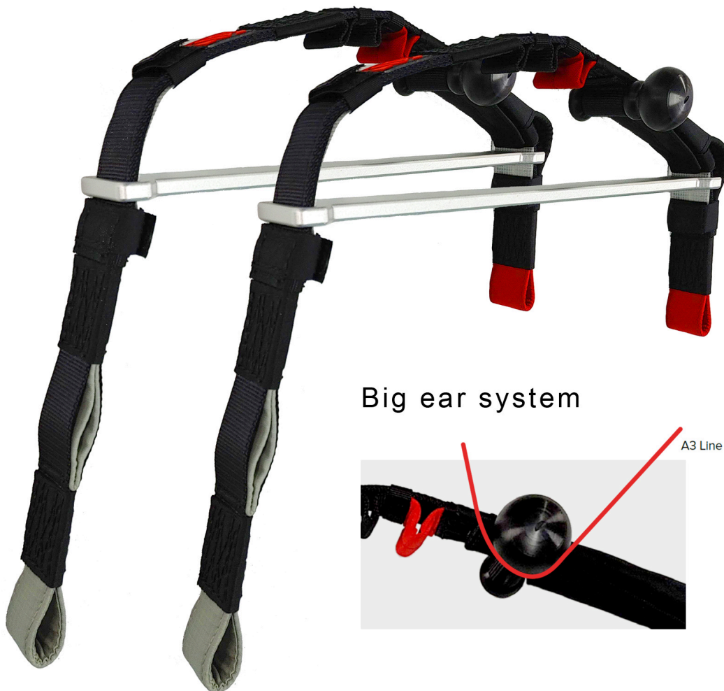
Figura: Separadores rígidos de 30mm para la Fuse mini
