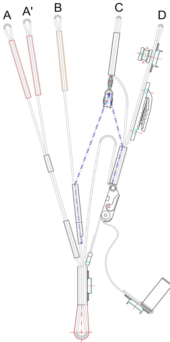
Figura: Bandas convencionales de 20 mm
